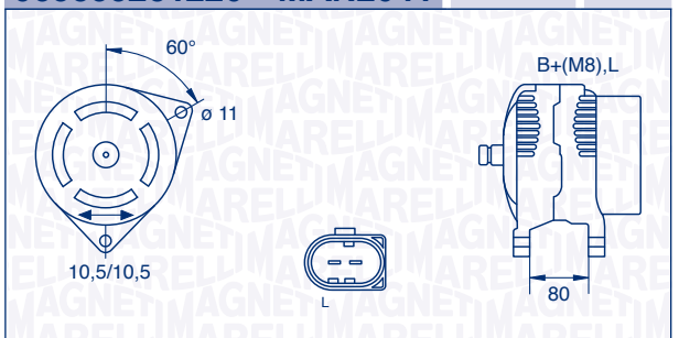
063533251220 – MAN2041 110 A 12 V
