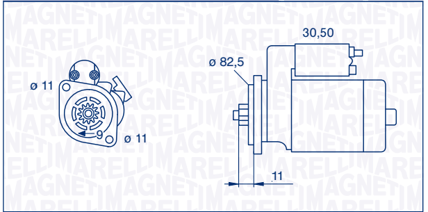
063280083010 – MSN8083 2,5 kW 12 V
