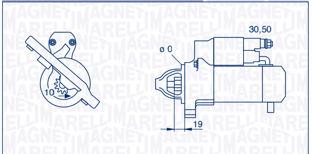
063280084010 – MSN8084 1,4 kW 12 V
