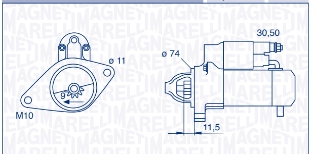
063280085010 – MSN8085 1,3 kW 12 V
