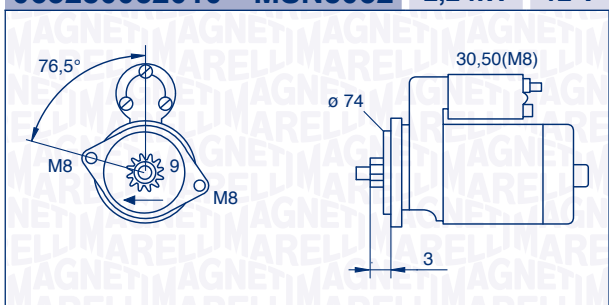
063280052010 – MSN8052 2,2 kW 12 V
