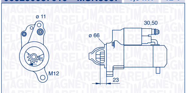
063280087010 – MSN8087 1,8 kW 12 V
