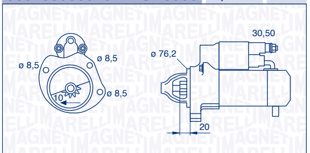
063280086010 – MSN8086 1,4 kW 12 V
