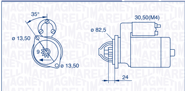
063523620760 – MSN2051 2,4 kW 12 V
